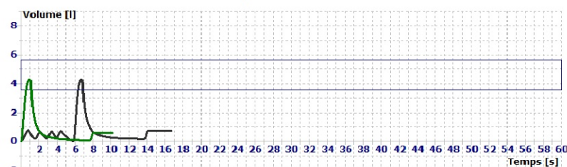
CVL Courbe Volume/Temps
